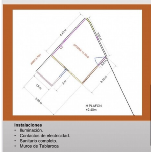
PLANO OFICINA
